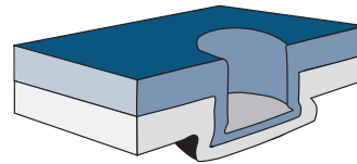
Best-Point-liitos ilman hitsausta
